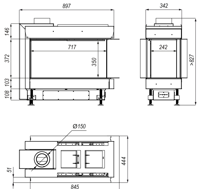
Rysunek 7. Wymiary DEFRO HOME VITAL 51 S U.
