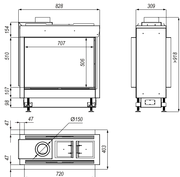
Rysunek 8. Wymiary DEFRO HOME VITAL 51 S T
