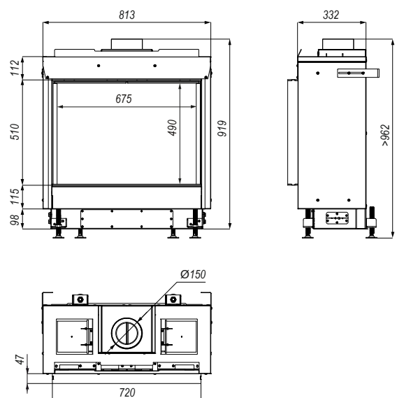
Rysunek 9. Wymiary DEFRO HOME VITAL 51 S.
