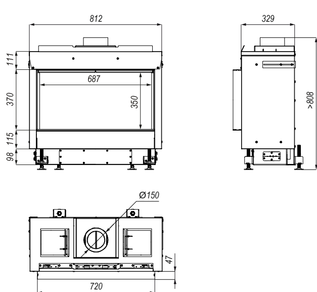
Rysunek 2. Wymiary DEFRO HOME VITAL 37 S.
