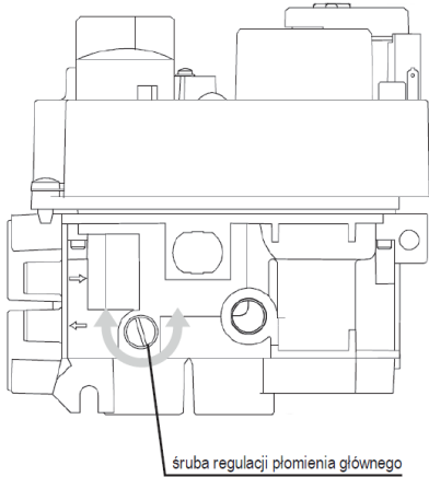
Rysunek 27. Położenie pokrętła zaworu głównego i umiejscowienie śruby regulacji płomienia głównego.
