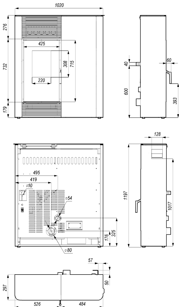
Výkres 3. Rozměry krbových kamen DEFRO HOME SLIMPELL.
