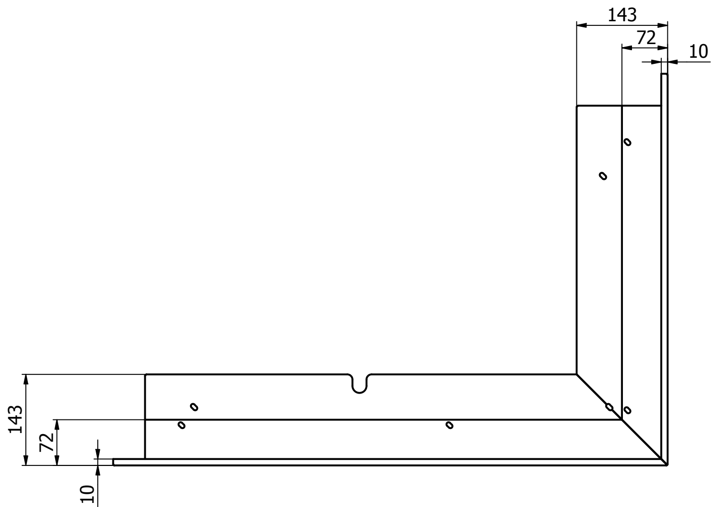
Maskownica 50 głęboka
